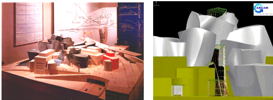
FIGURA 2: Modelo físico e digital do Museu Guggenheim de Bilbao (SPERLING, 2008)
